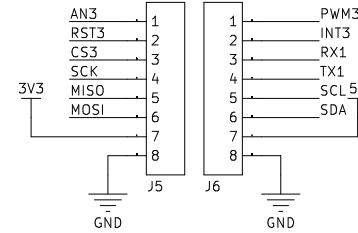
MikroBUS3
