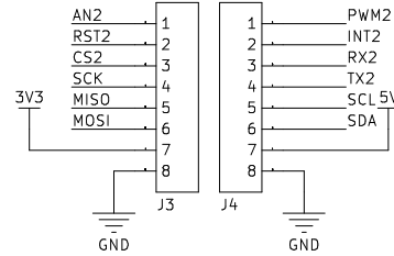
MikroBUS2
