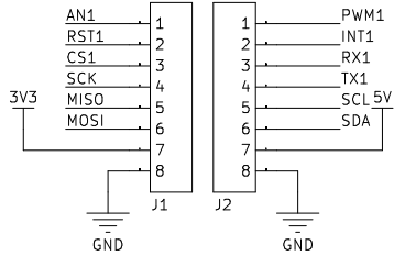
MikroBUS1
